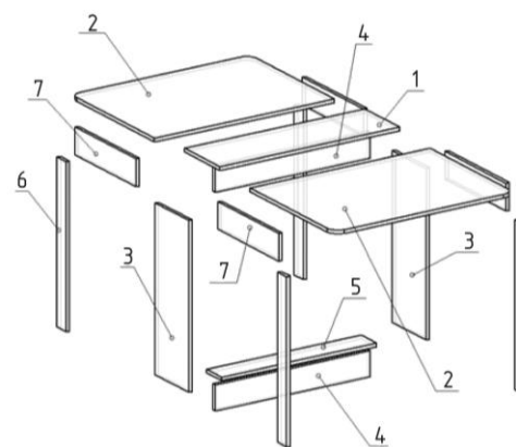
Рисунок 1 – Схема сборки
