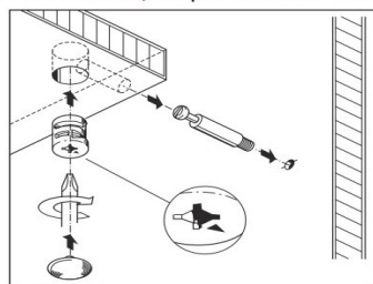
Монтаж эксцентриковой стяжки
