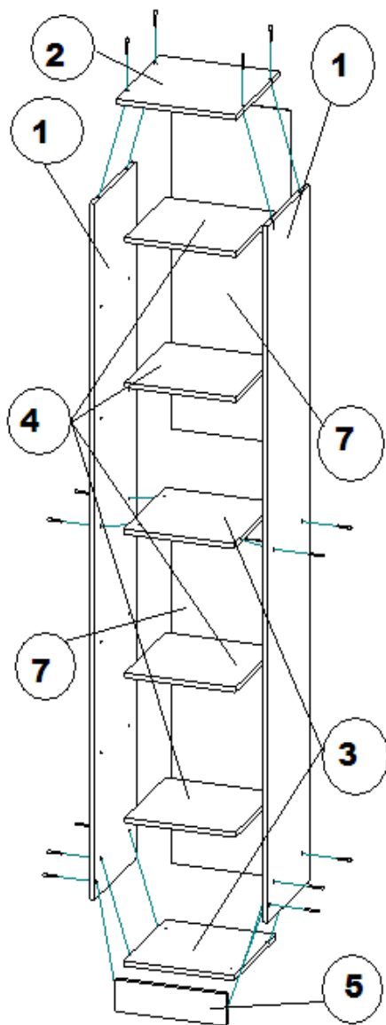
Рисунок 1 — схема сборки
